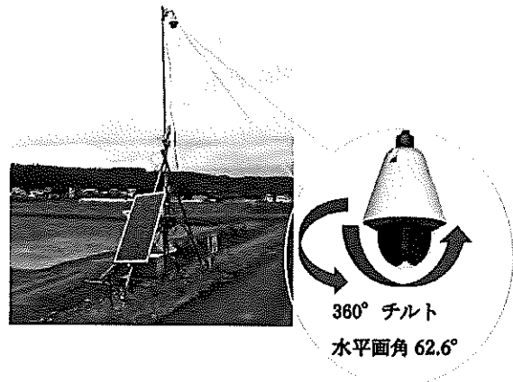
IOTカメラ・ソーラー発電設置状況
