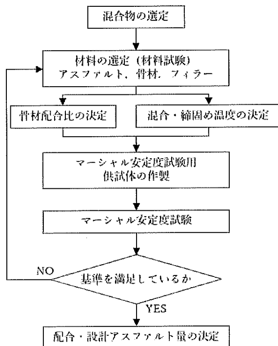
図-2 配合設計手順 2) を引用、簡略化
