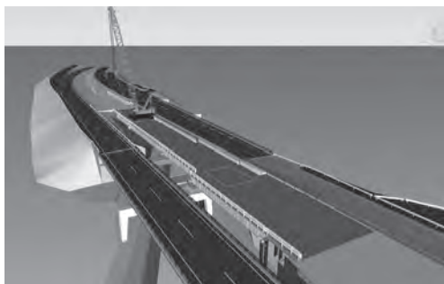
図-6 3次元モデル(仮橋設置)
