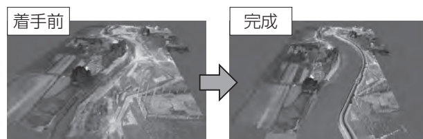
図-8 点群地形データと3次元モデル
