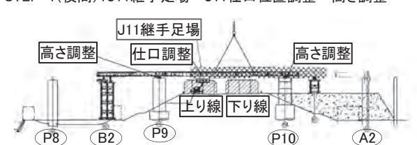
図-4 架設ステップ図
