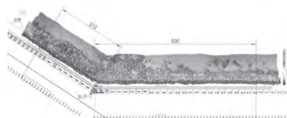
図-5 深浅鳥観図
