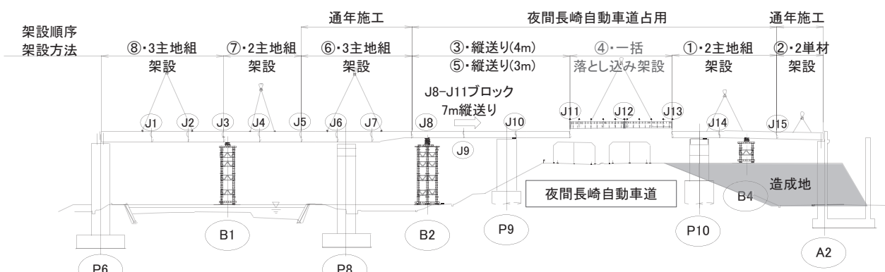
図－3 架設計画図（変更後）
