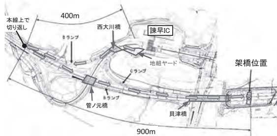
図－2 地組桁輸送経路図
