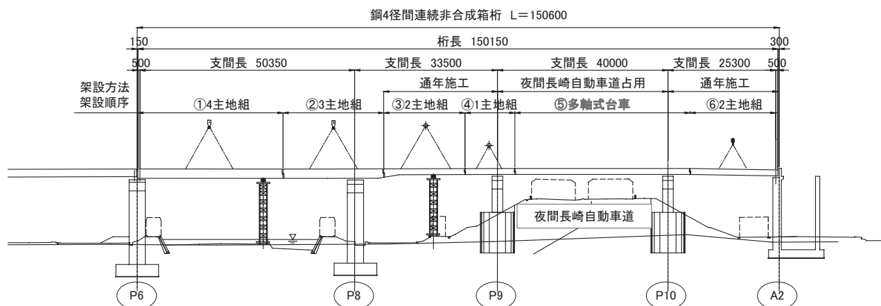
図－1 架設計画図 (当初計画)
