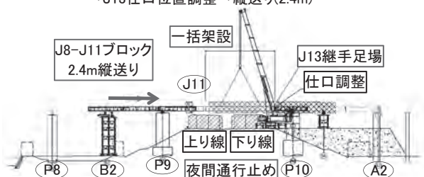
STEP-2(夜間): J11-J13架設→J13継手足場 →J13仕口位置調整→縦送り(2.4m)
