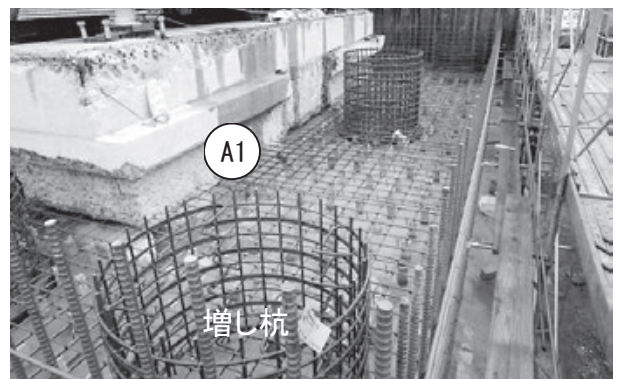
図-10 ⑥, ⑧増し杭、底版増築
