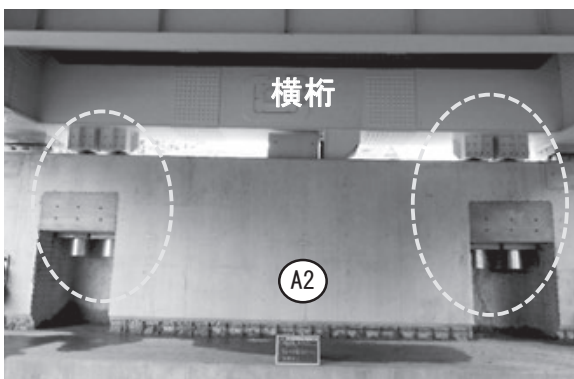
図-9 ⑨負反力対策工 PCケーブル設置
