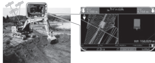
図-10 3D-MGバックホウでの作業状況
