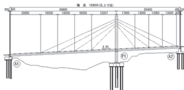
図-2 橋梁一般図
