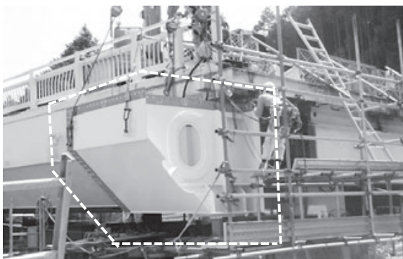
図-7 ⑤部分取替えによる主桁補修
