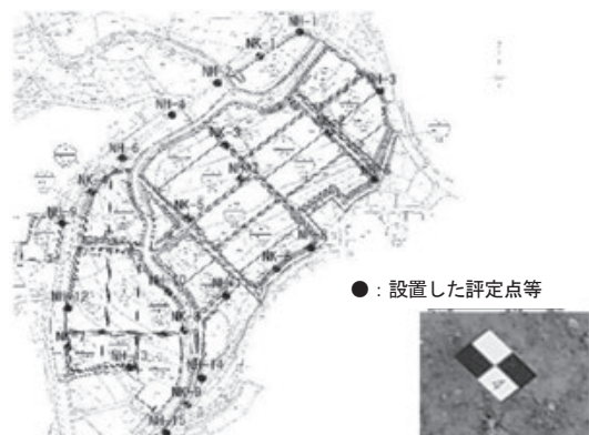
図-6 評定・検証点設置計画
