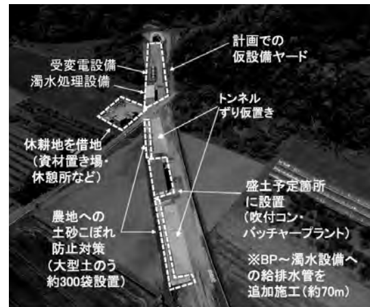
図-8 仮設備設置状況
